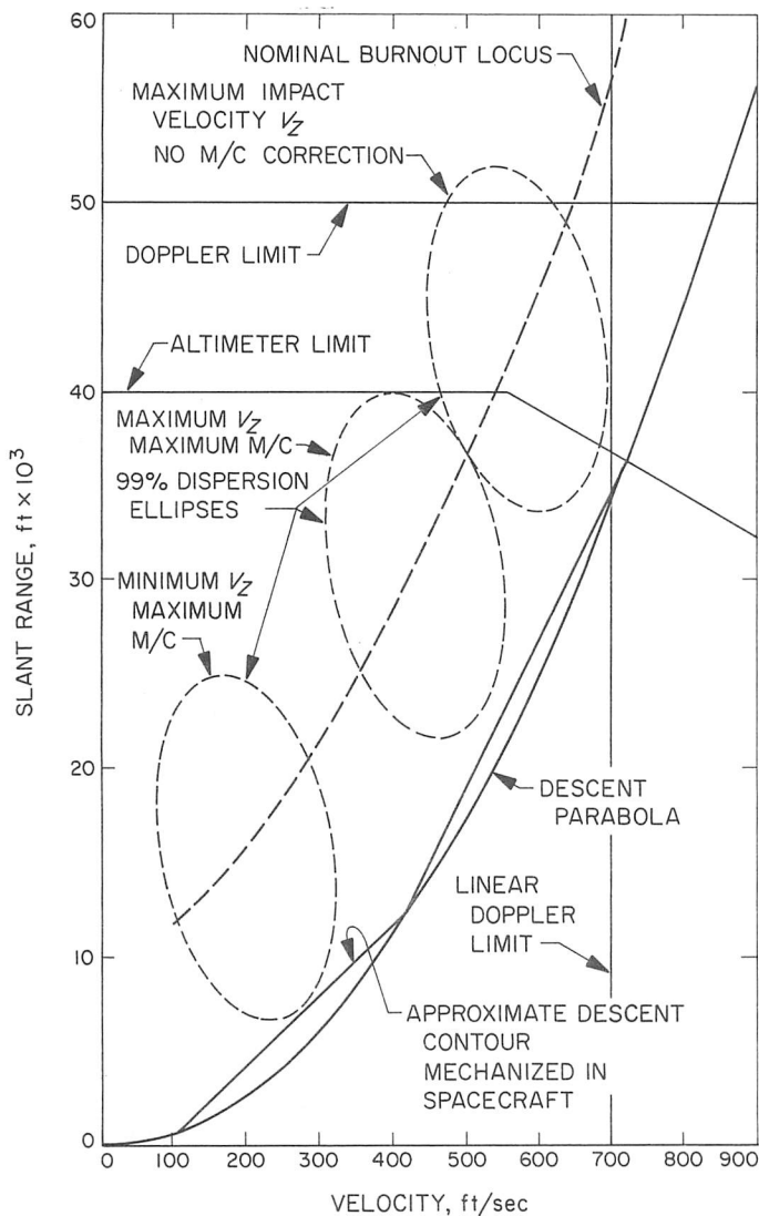
Fig. IV-7. Range-velocity diagram
