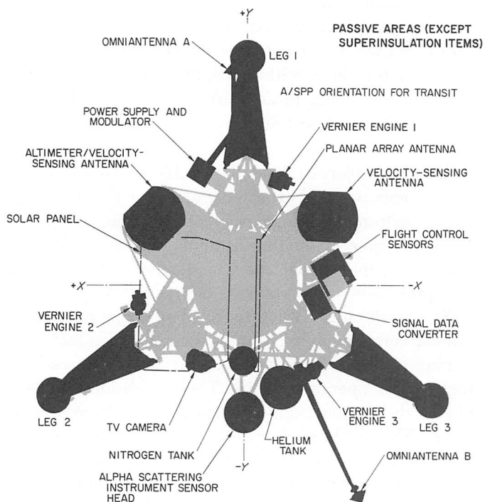
Fig. IV-17. Thermal design
