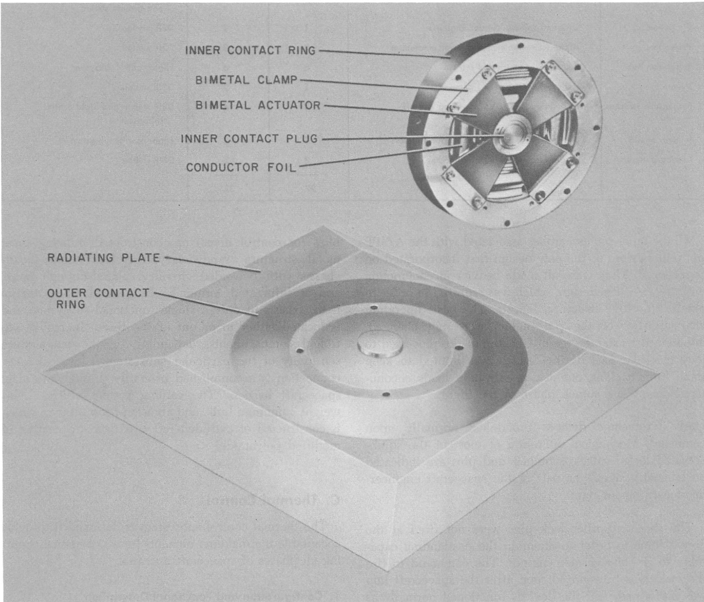
Fig. IV-16. Thermal switch
