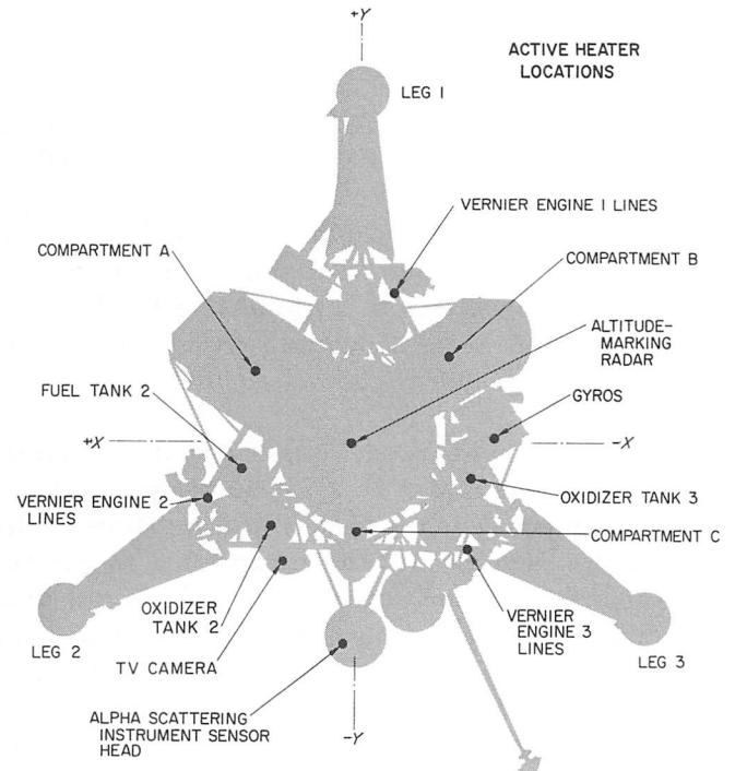
Fig. IV-17. Thermal design
