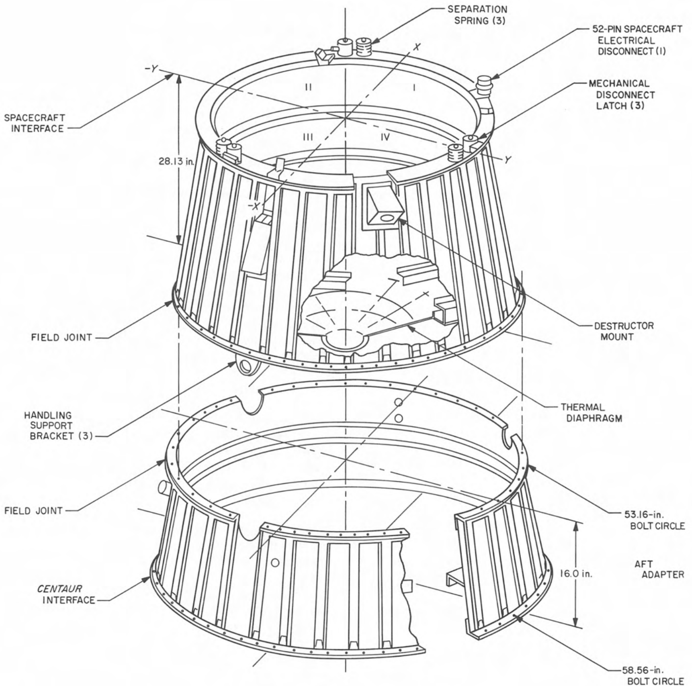
Fig. VIII-11. Centaur/Surveyor adapter
