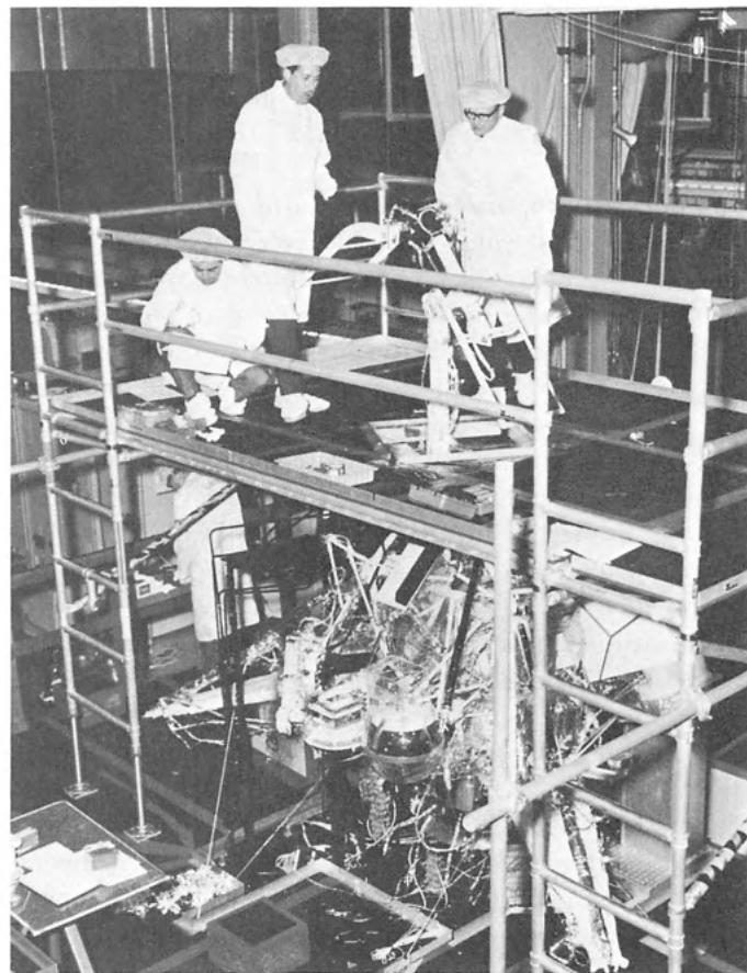
Fig. IX-4. STEA high access stand
