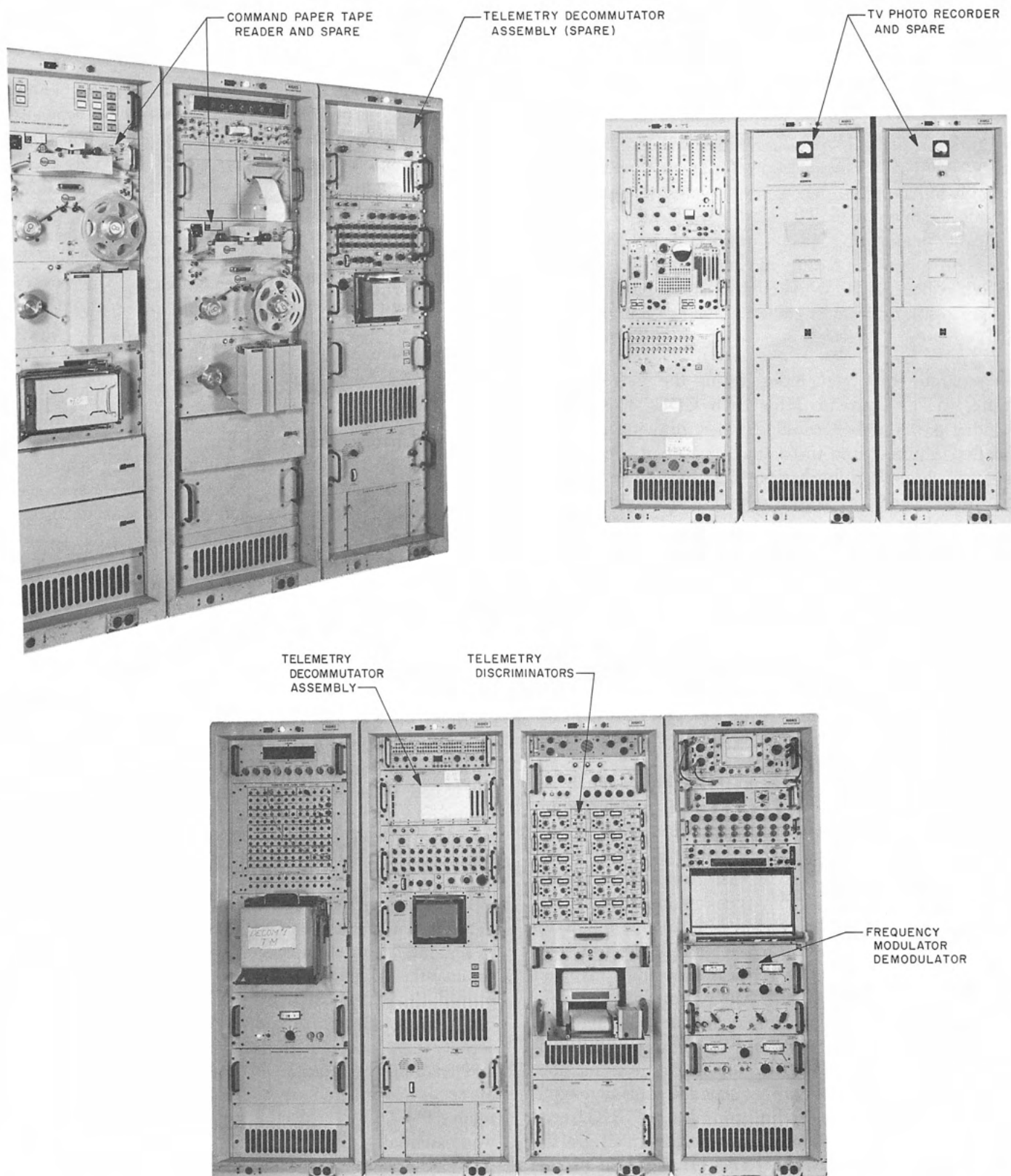
Fig. VII-4. The CDC equipment for DSIF
