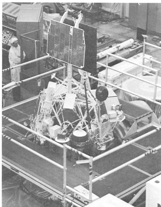
Fig. XI-14. Vibration test setup
