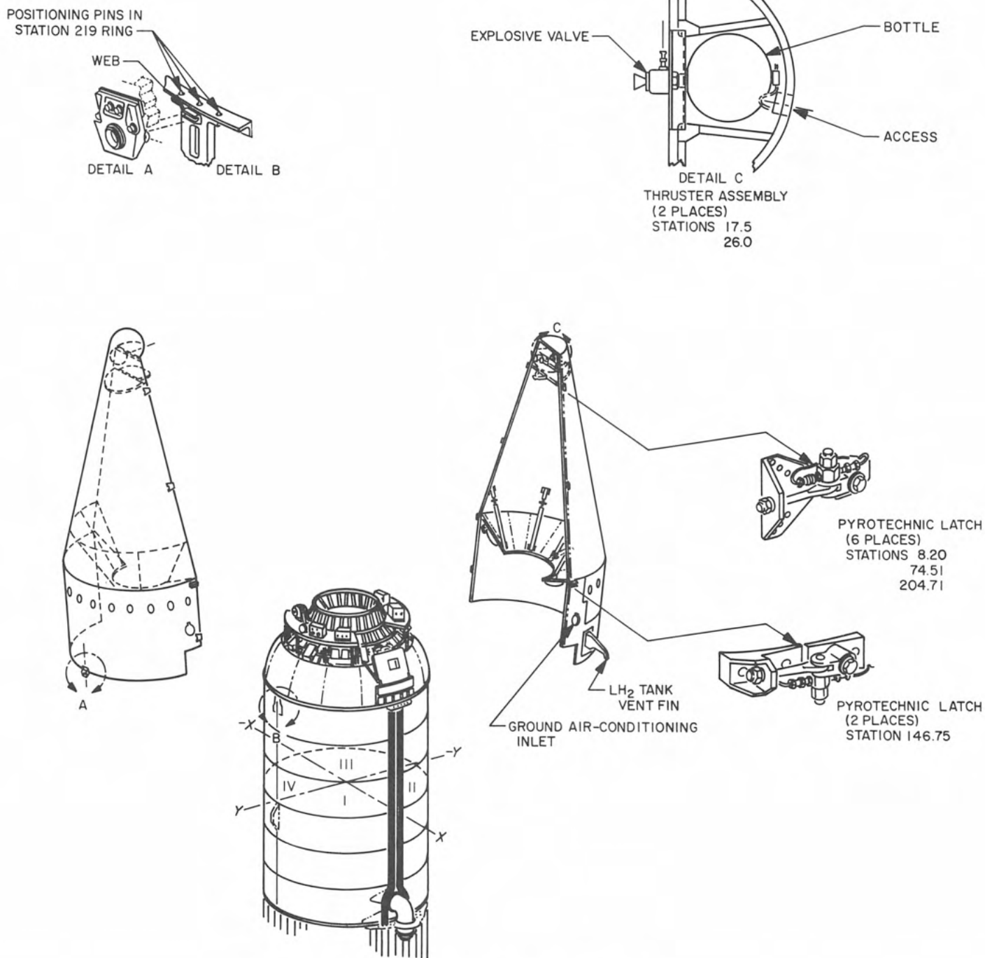
Fig. VIII-9. Nose fairing jettison system
