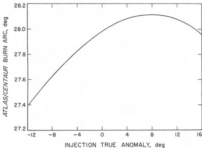
Fig. VI-6. Direct-ascent burn arc
