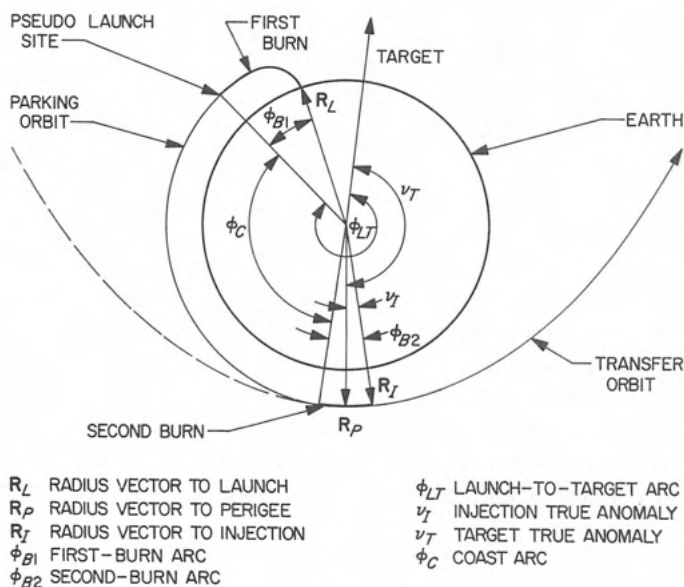
Fig. VI-8. In-plane parking-orbit ascent geometry
