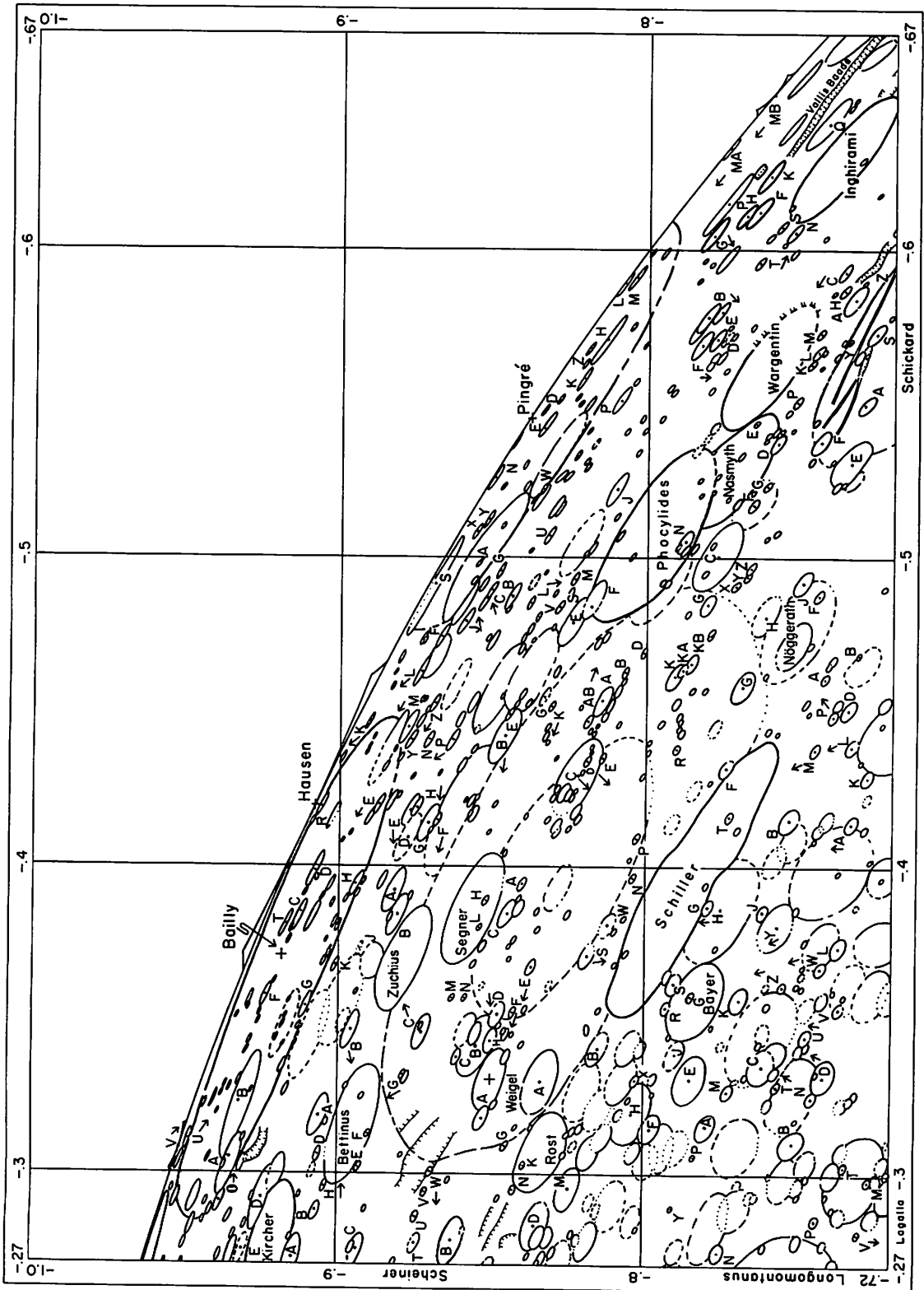
LUNAR NOMENCLATURE
