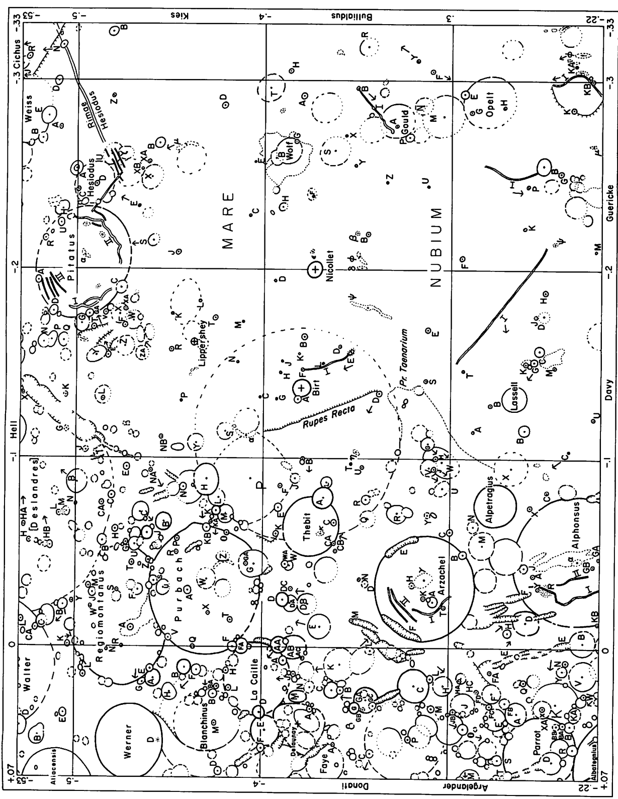
LUNAR NOMENCLATURE
